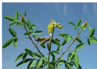
C. micans
